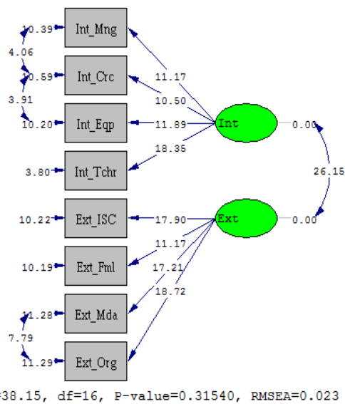
شکل ۲. مدل ساختاری پژوهش در حالت معناداری ضرایب
